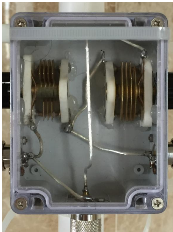
图 12 “Army Loop”小环天线调谐及匹配电容盒
