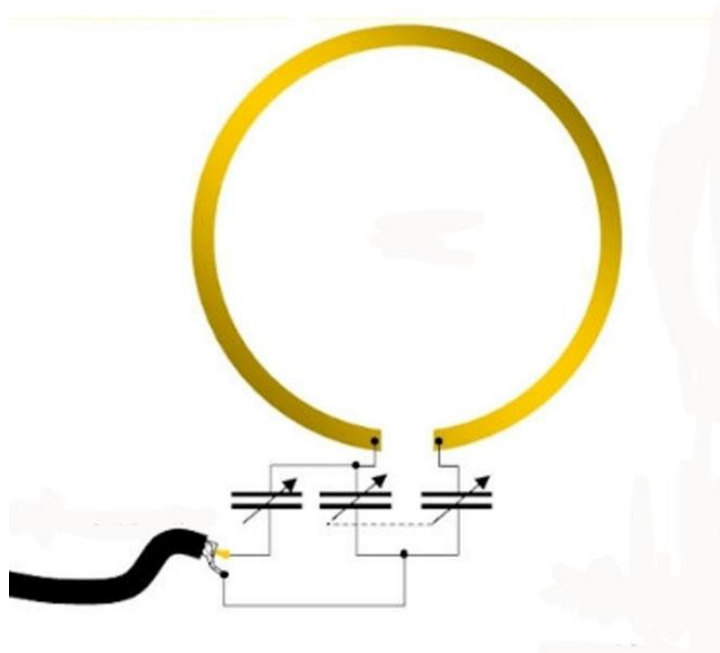
图 9 军用环（Army Loop）
