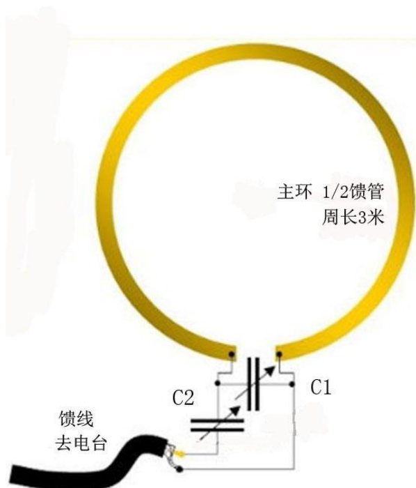
图 10 简化的“军用环”小环天线电路
