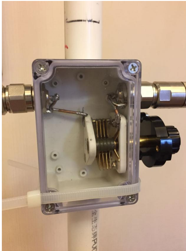
图 3 电容盒
