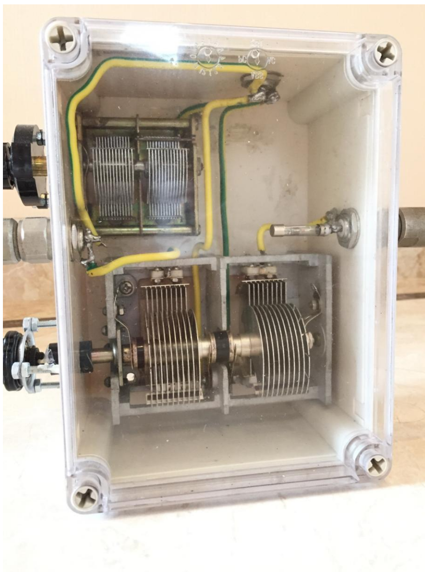
军用环的调谐与匹配电容盒
