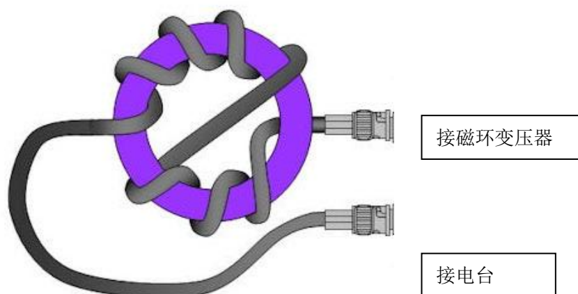
图 5 巴伦绕法
