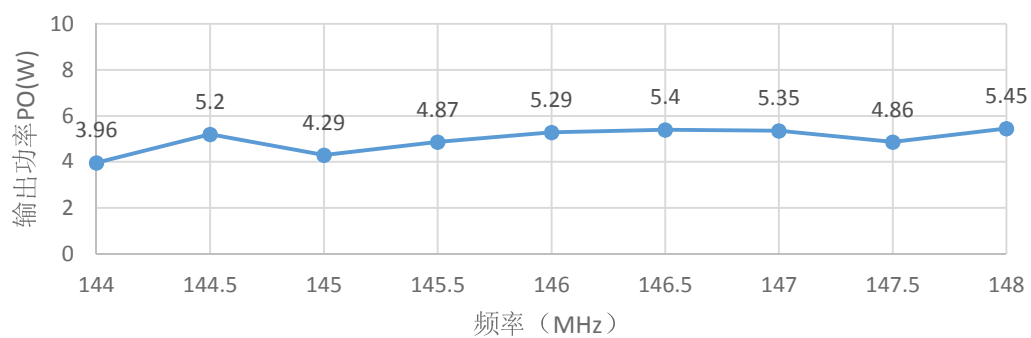
2米功率测试（144M~148M）
