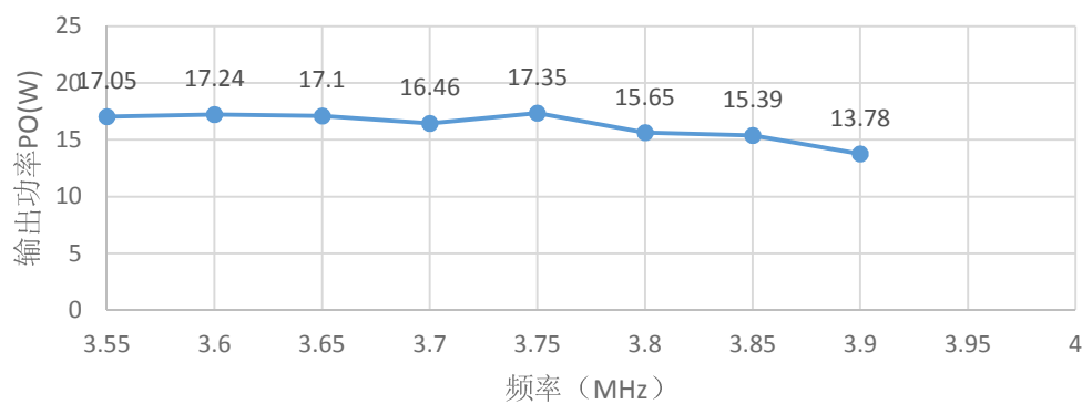
80米功率测试（3.5M~3.9M）
