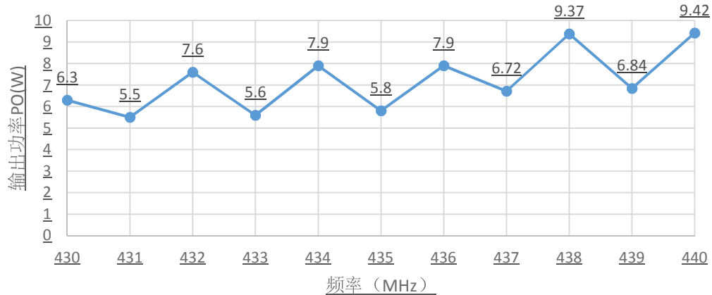
0.7米功率测试（430M~440M）
