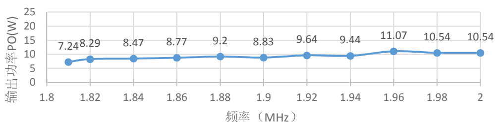
160米功率测试（1.8M~2.0M）
