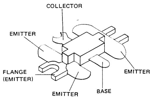
2SC2539
