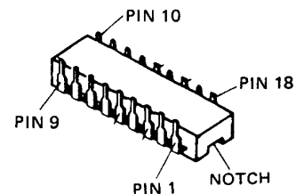
TC9122
