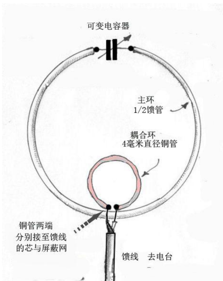
图 6 用耦合环馈电的小环天线电气连接图
