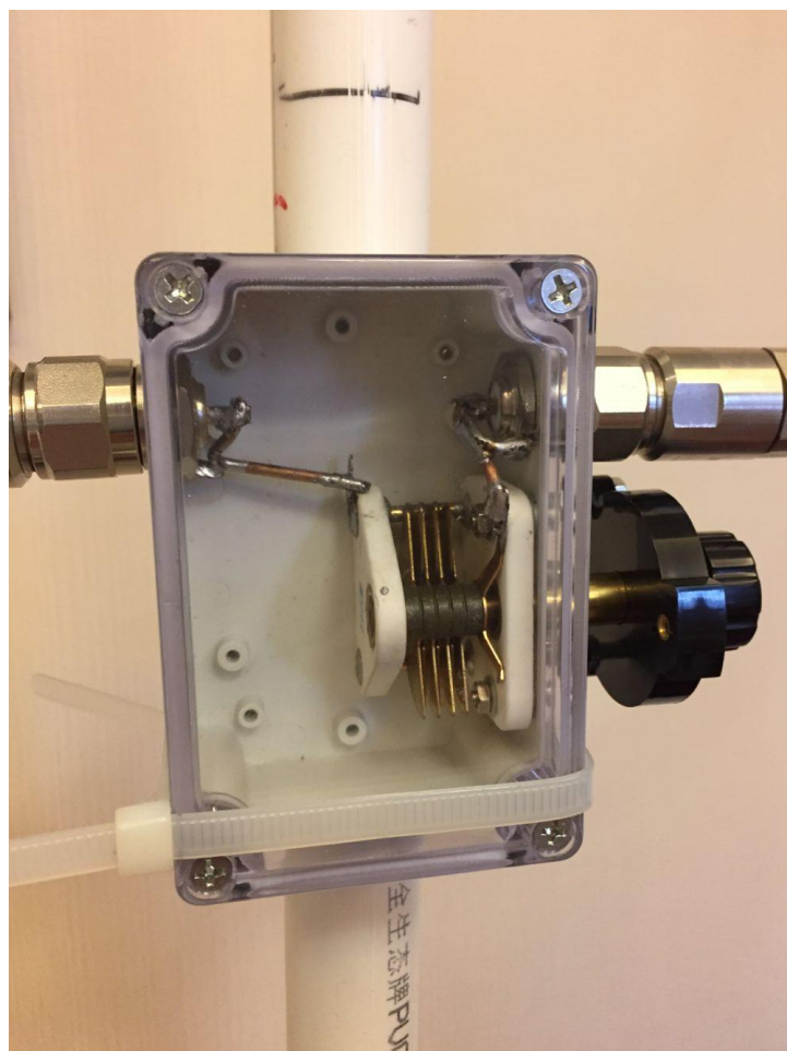
图 3 电容盒
